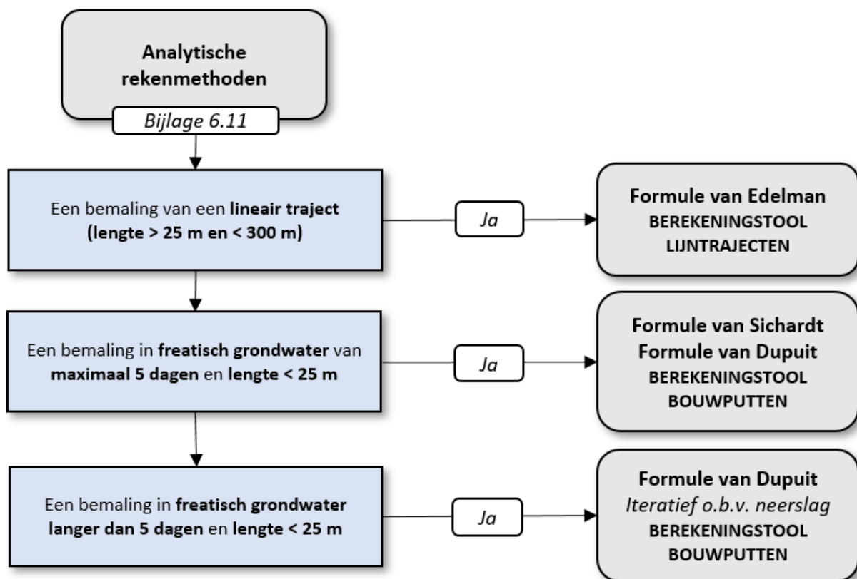
Figuur 7: Stroomschema ter bepaling van de toe te passen analytische rekenformule.
