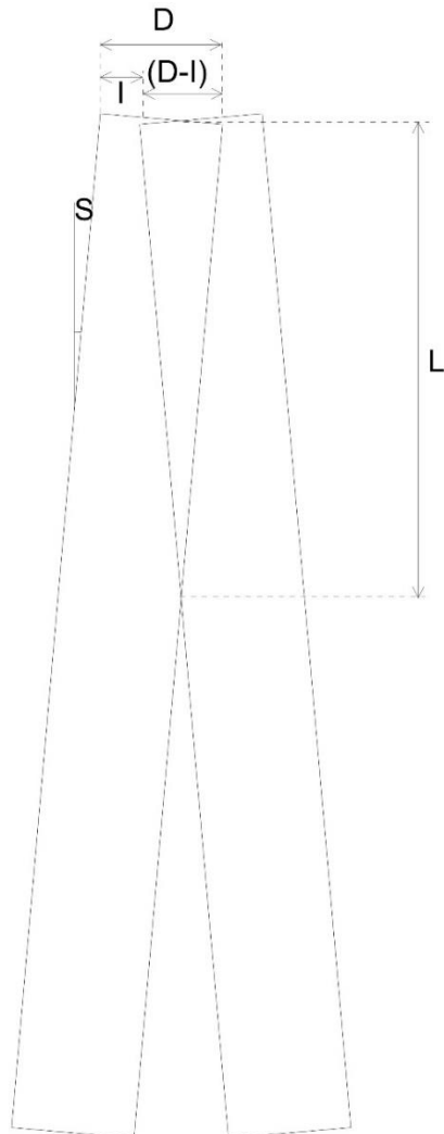
Figuur 70 visuele voorstelling parameters voor berekening L
