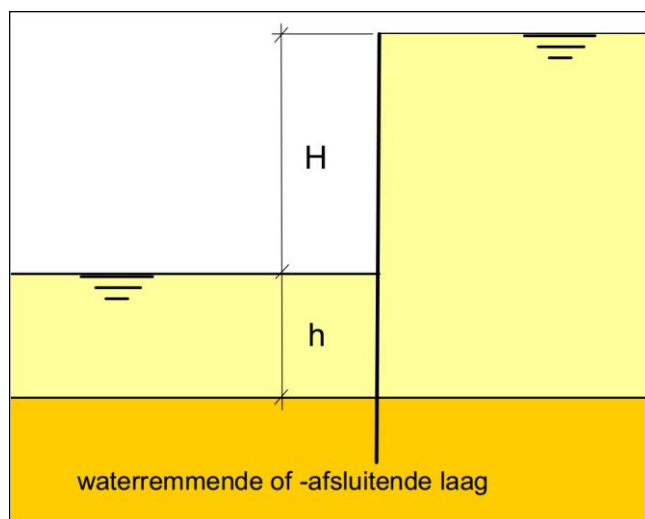
Figuur 66 opstelling waterkerende wand
