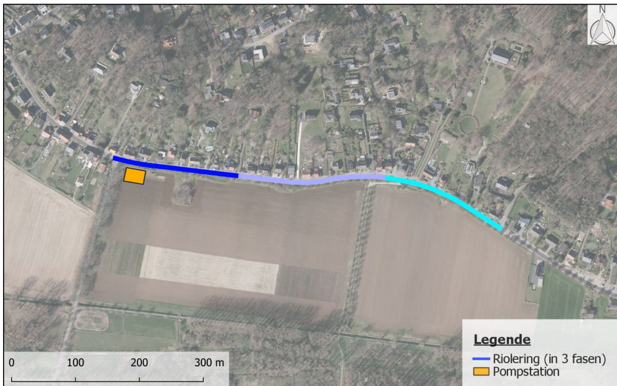
Figuur 9: Fictief voorbeeld van de aanleg van een pompstation en de heraanleg van het rioleringsstelsel (bemaling in 3 fasen) in de aangrenzende straat.
