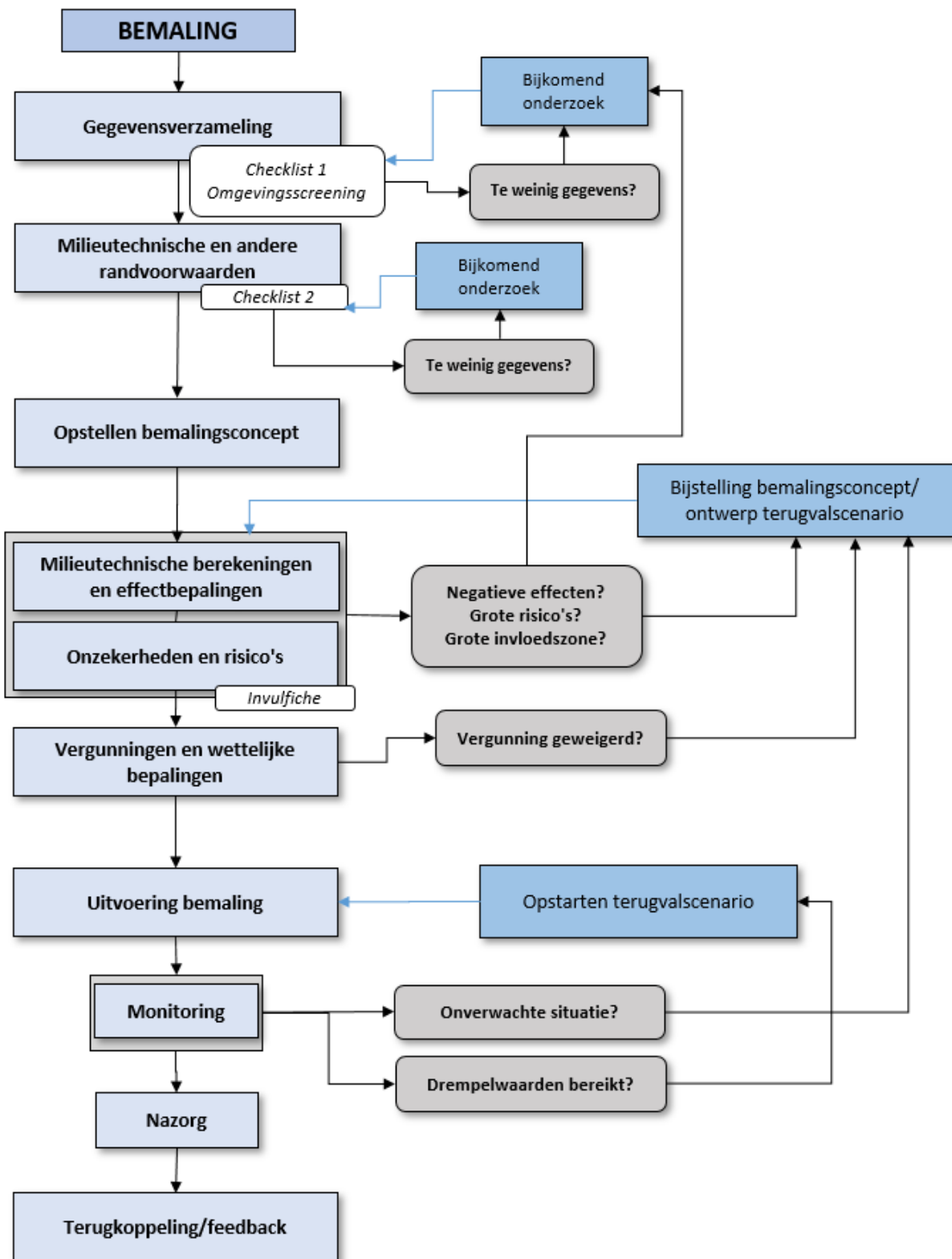
Figuur 1: Stappenplan te volgen bij het opstellen van een bemalingsstudie en het uitvoeren van de bemaling. De belangrijke onderdelen monitoring, nazorg en terugvalsscenario moeten reeds in de bemalingsstudie behandeld worden.
