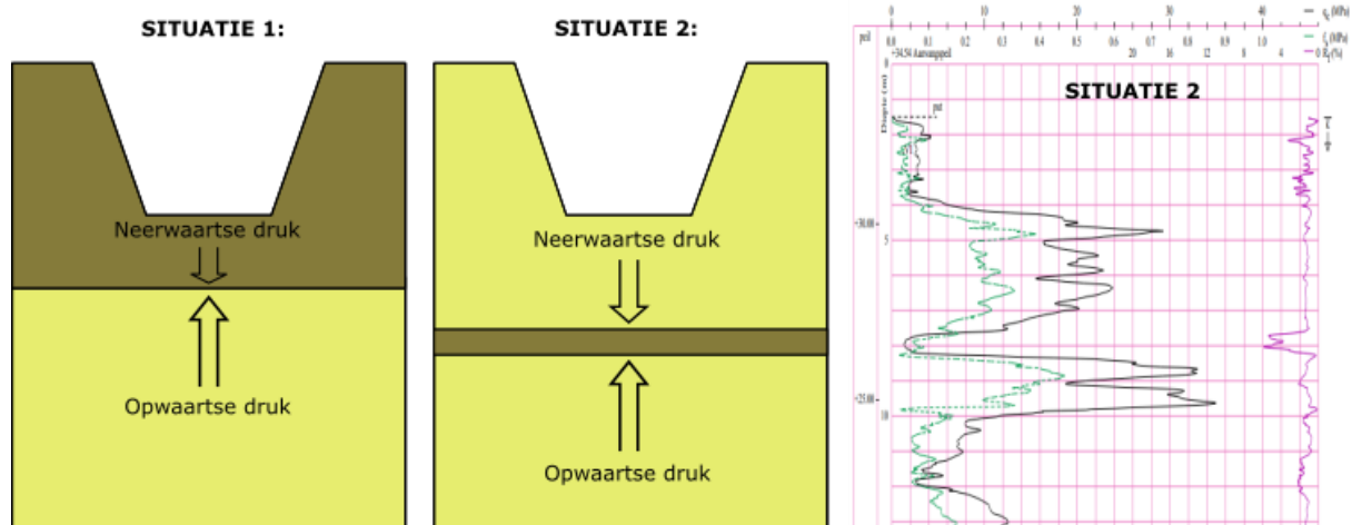
Figuur 2: Illustratie van het opbarstgevaar bij een situatie waarbij uitgegraven wordt in een waterremmende laag (situatie 1) en een situatie waarbij uitgegraven wordt tot op een zekere diepte boven een waterremmende laag (situatie 2 met voorbeeld sondering).
