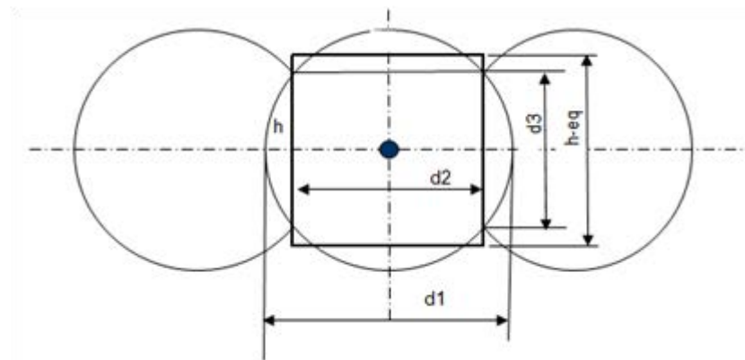
Figuur 67 wand bestaande uit snijdende kolommen
