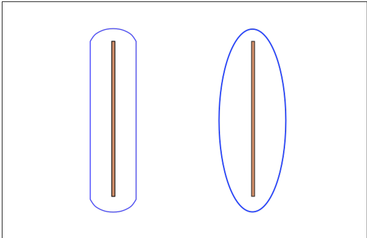
Figuur 6: conceptuele vergelijking tussen de invloedsstraal voor de bemaling van een sleuf berekend door middel van de Formule van Edelman (links) en gesimuleerd in een grondwatermodel (rechts).
