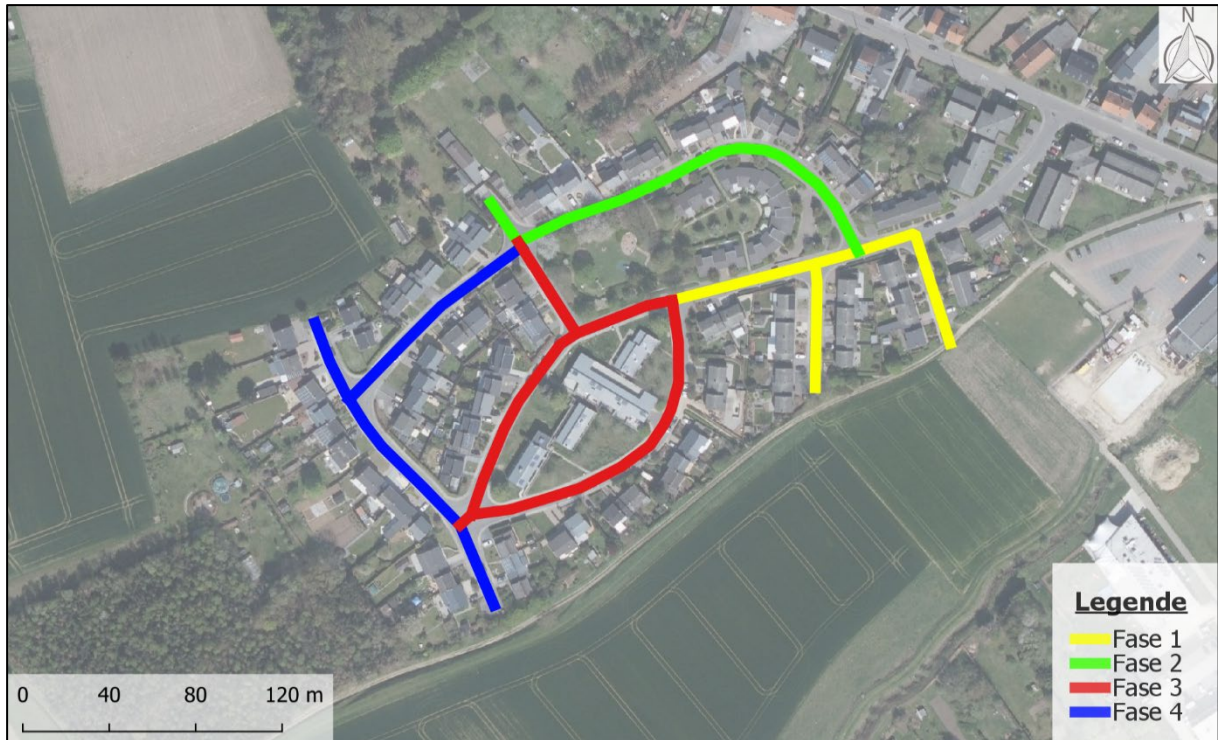
Figuur 8: Fictief voorbeeld van de heraanleg van wegenis en rioleringen in een woonwijk. De werken, en dus ook de bemalingen, worden uitgevoerd in 4 fasen. Deze fasen kunnen gemeld/vergund worden als aparte deeltrajecten indien de bemalingen elkaar niet beïnvloeden in tijd en ruimte.
